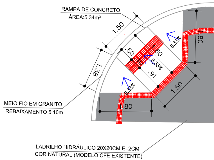
DETALHAMENTO DA RAMP RE1 ESCALA 1:75
