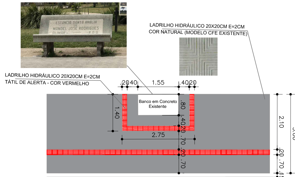
DETALHAMENTO DA CALÇADA E BANCOS ESCALA 1:75
