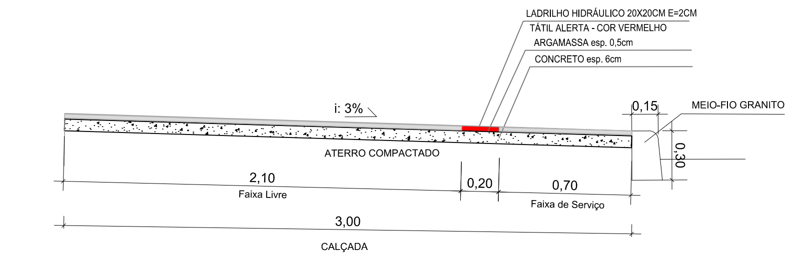
CORTE DA CALÇADA ESCALA 1:20
