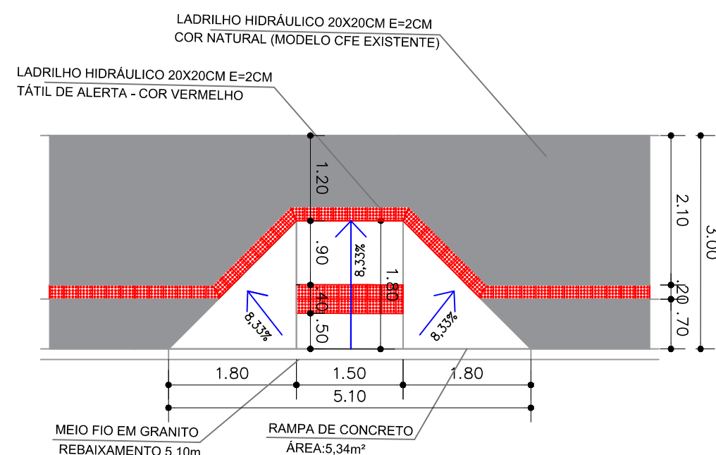
DETALHAMENTO DAS RAMPAS R01 À R07 ESCALA 1:75
