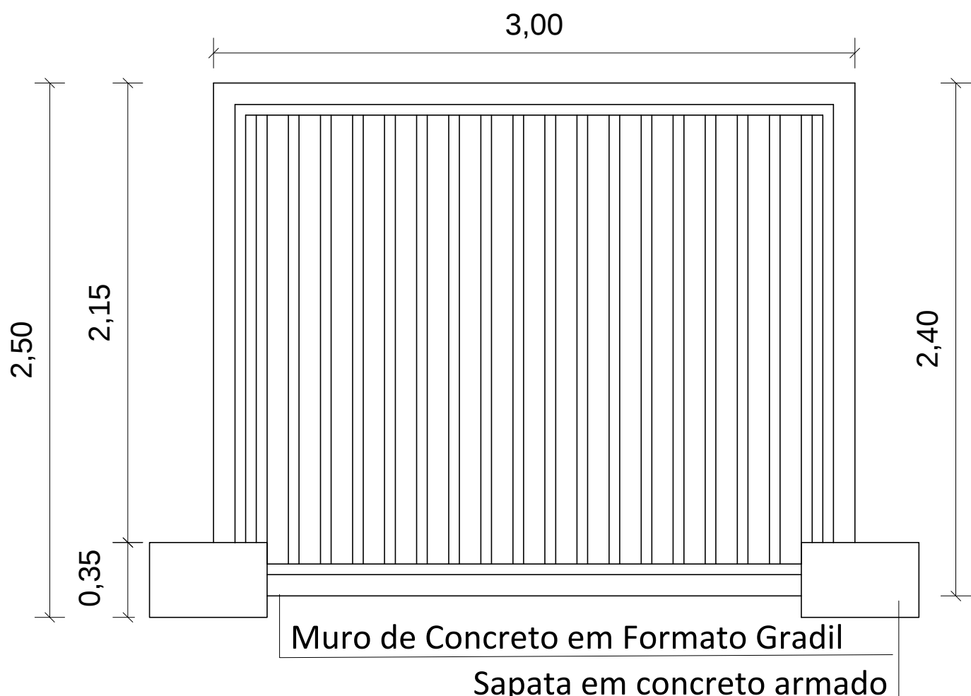
DETALHE MURO EM GRADIL ESCALA 1:25
