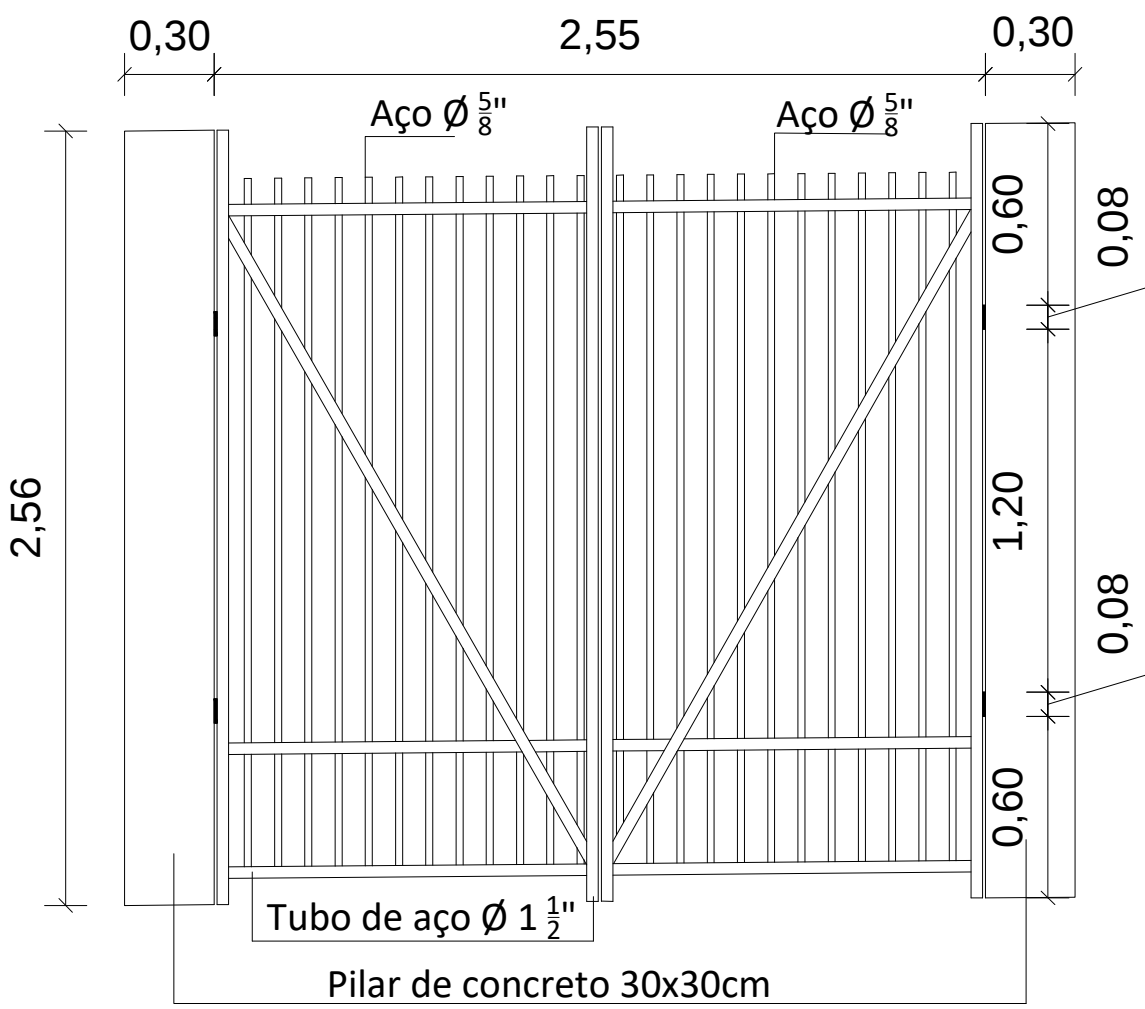
DETALHE PORTÃO 1 ESCALA 1:25
