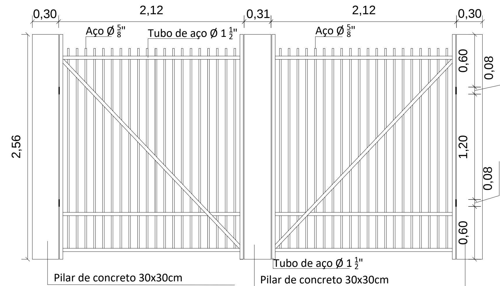
DETALHE PORTÃO 3 ESCALA 1:25
