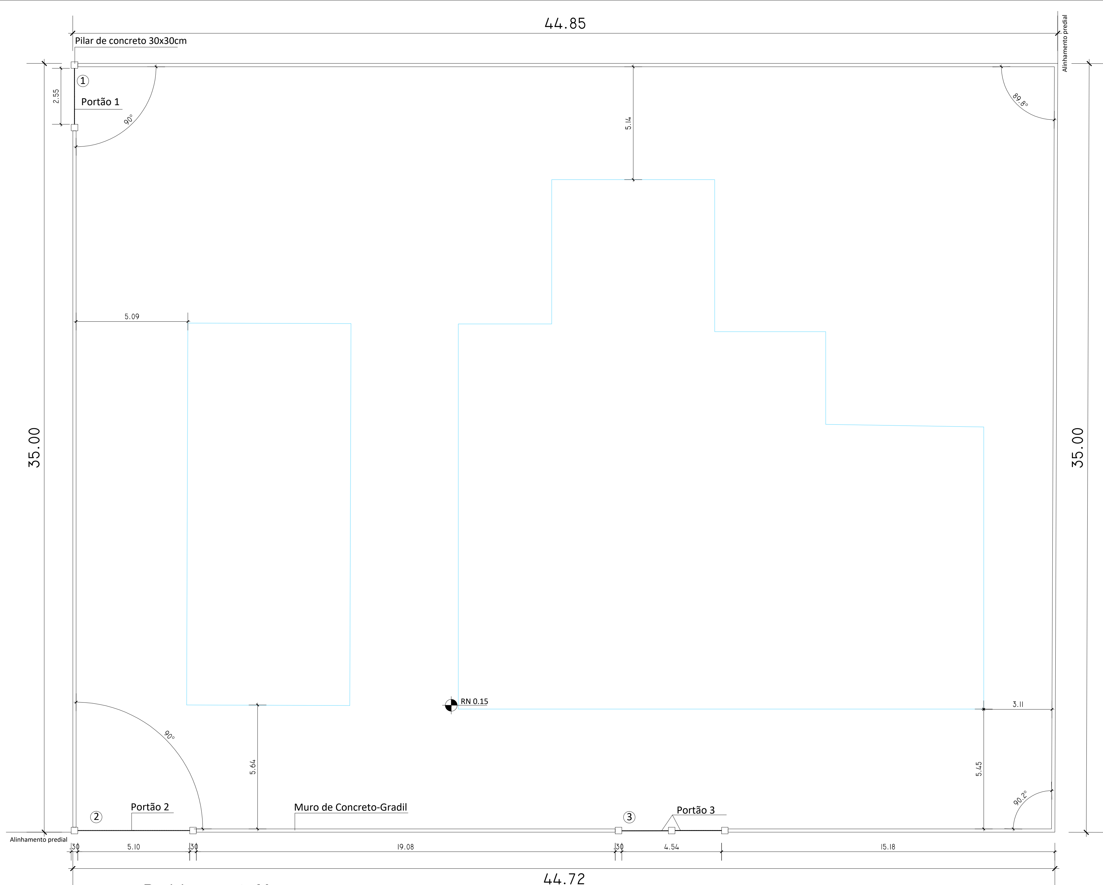
Posicionamento Muro ESCALA 1:100
