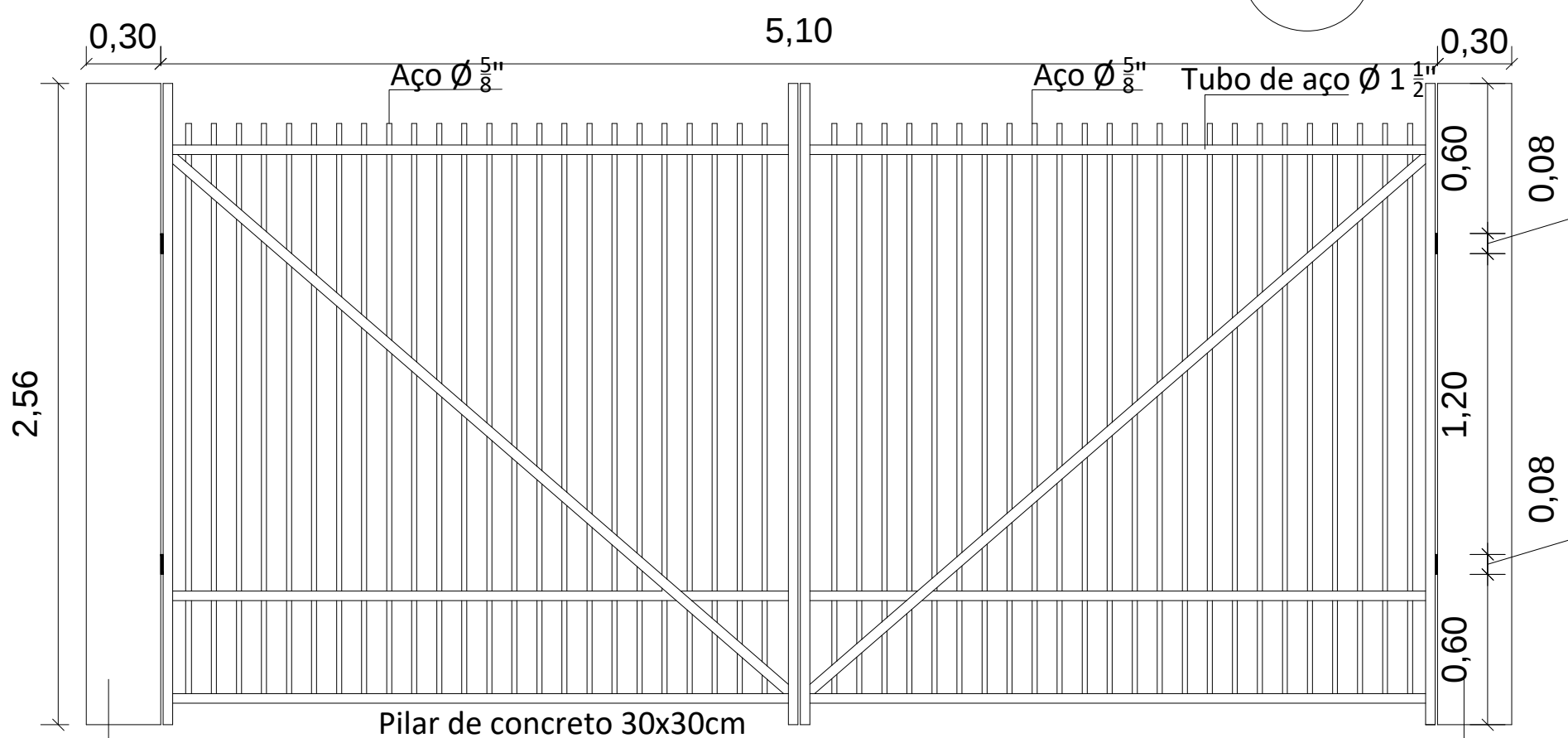
DETALHE PORTÃO 2 ESCALA 1:25
