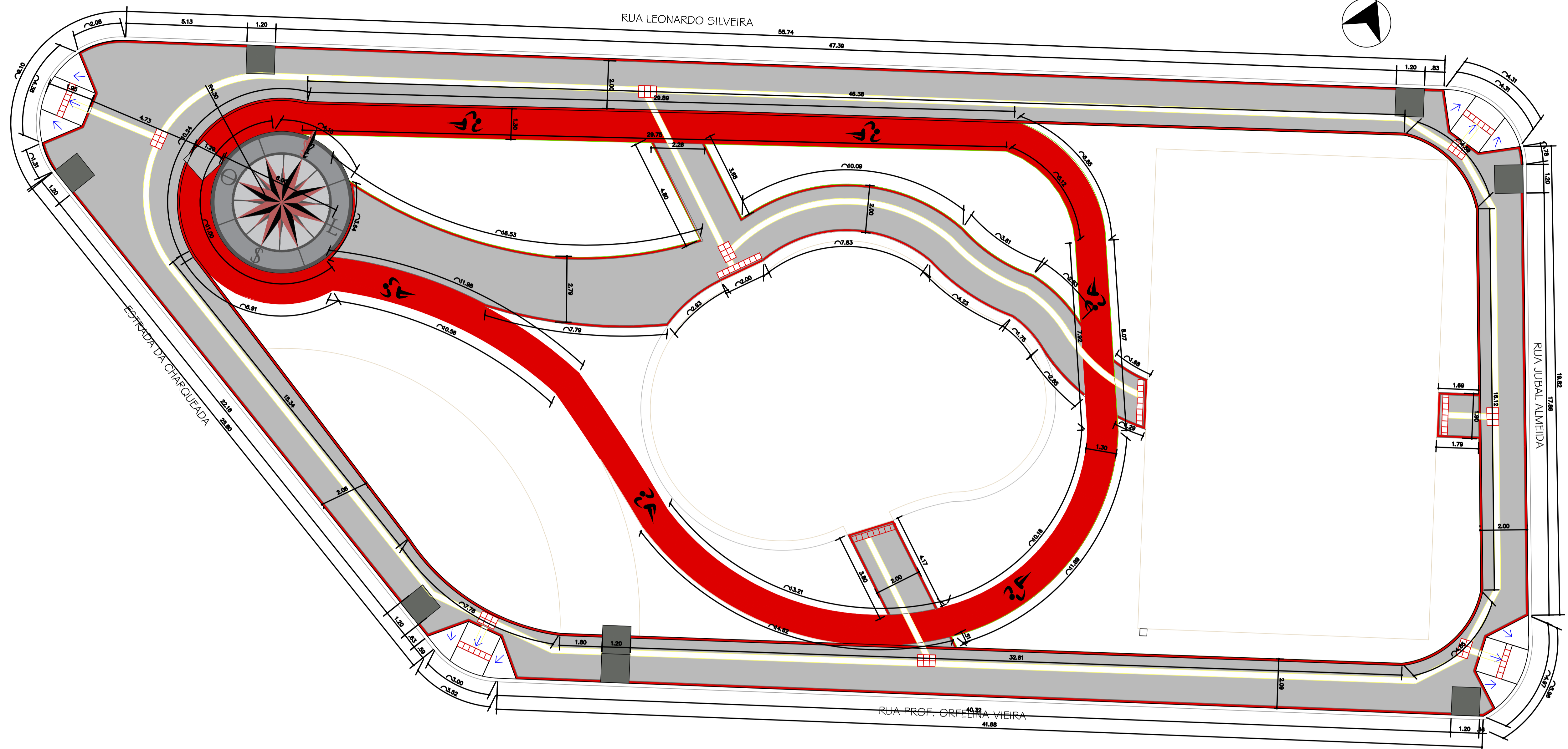
IMPLANTAÇÃO ESC: 1:100
