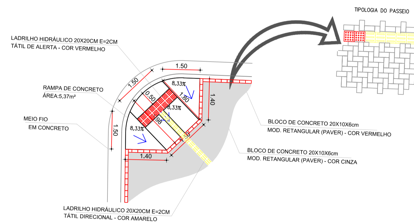
RAMPA ACESSÍVEL - NBR9050 ESC: 1:75
