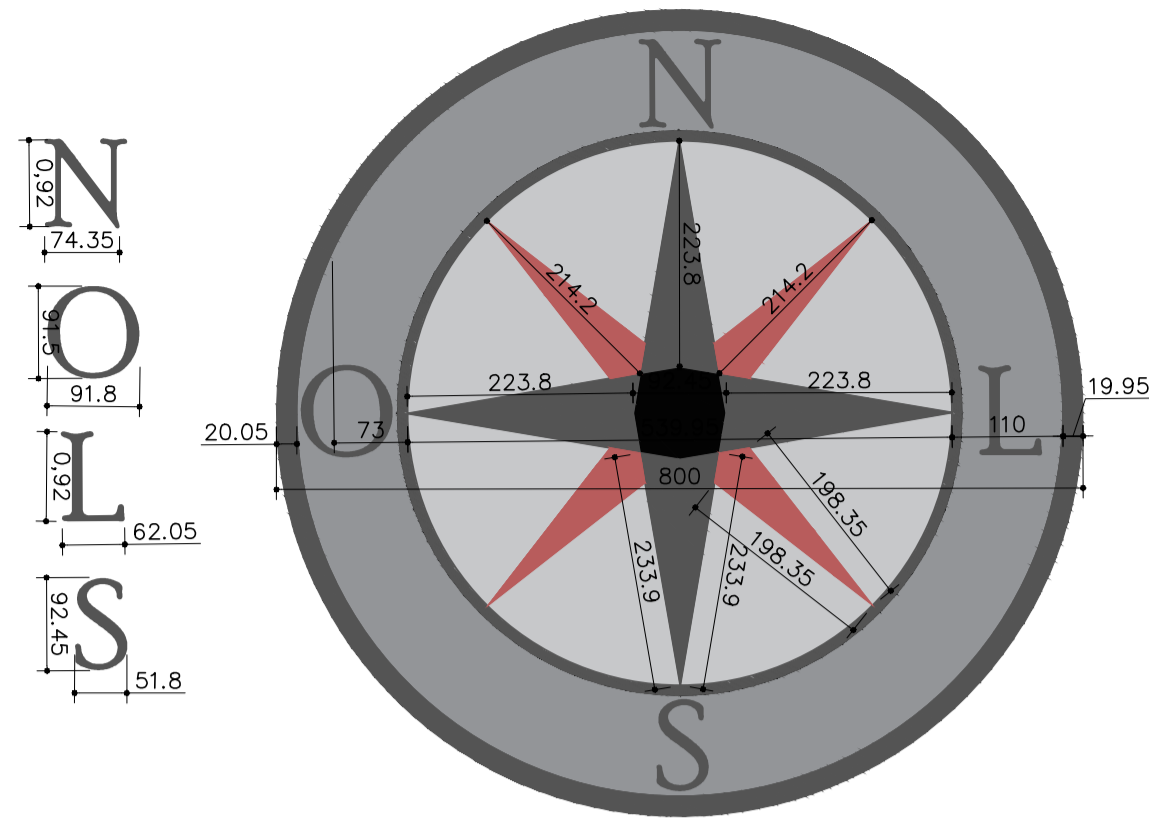
DETALHAMENTO ROSA DOS VENTOS ESC: 1:75
