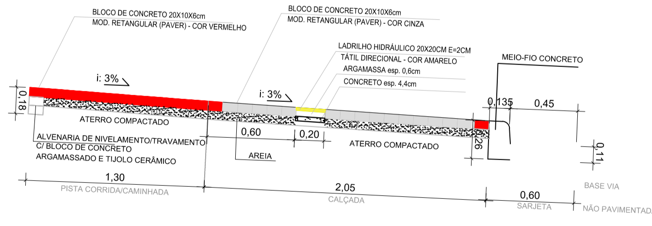
CORTE CALÇADA EXTERNA E PISTA DE CAMINHADA ESC: 1:25
