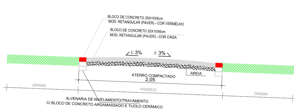
CORTE CALÇADA INTERNA ESC: 1:25
