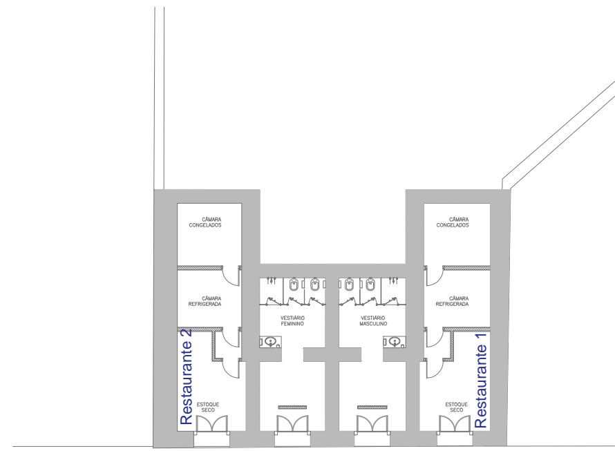
Planta Baixa Porão S/E
