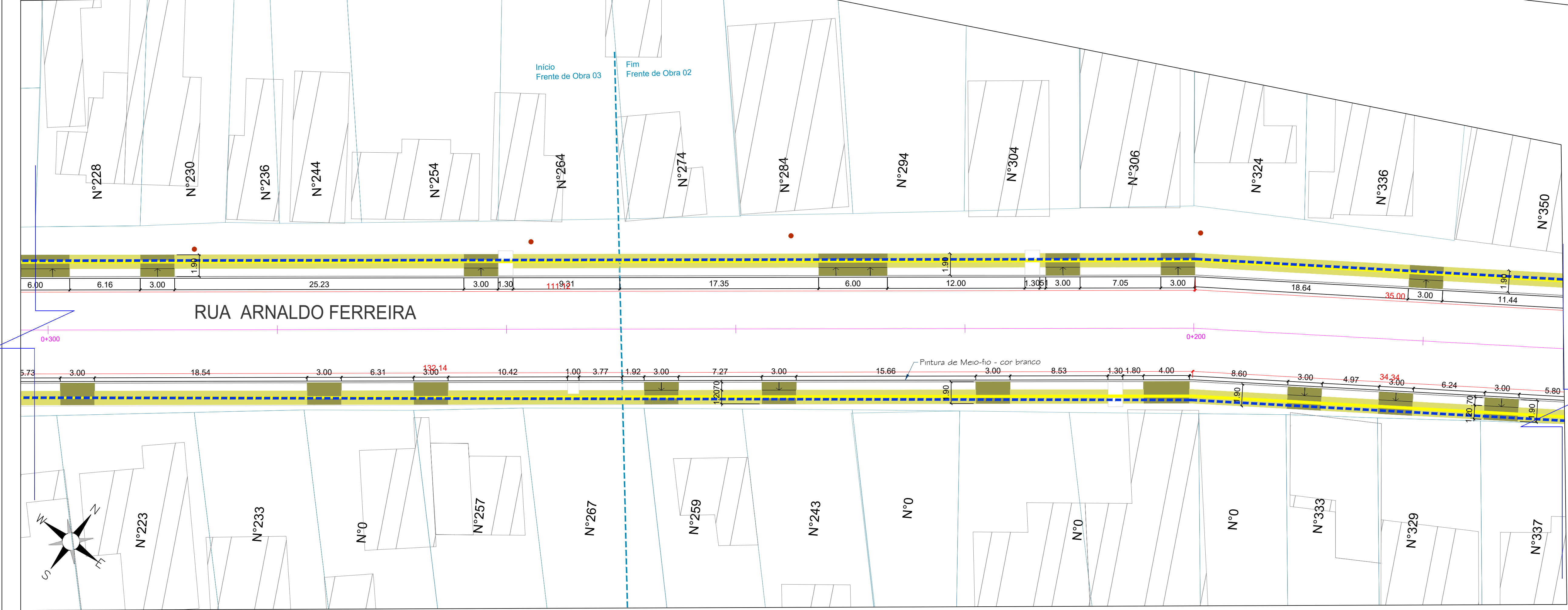
PROJETO ACESSIBILIDADE - - Rua Arnaldo Ferreira - km 0+170ao km 0+300 Escala 1:200
