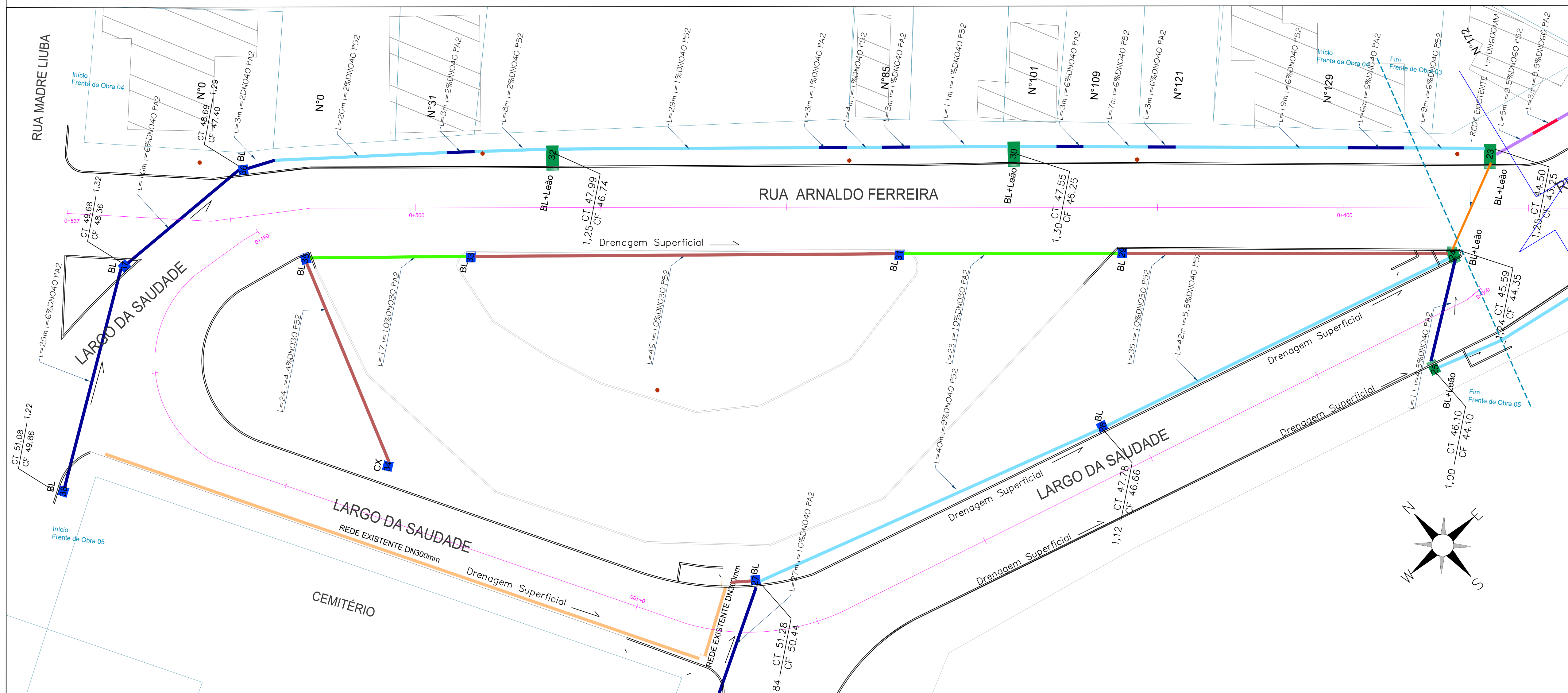
PROJETO DRENAGEM - - Rua Arnaldo Ferreira - km 0+380 ao km 0+537 Escala 1:250
