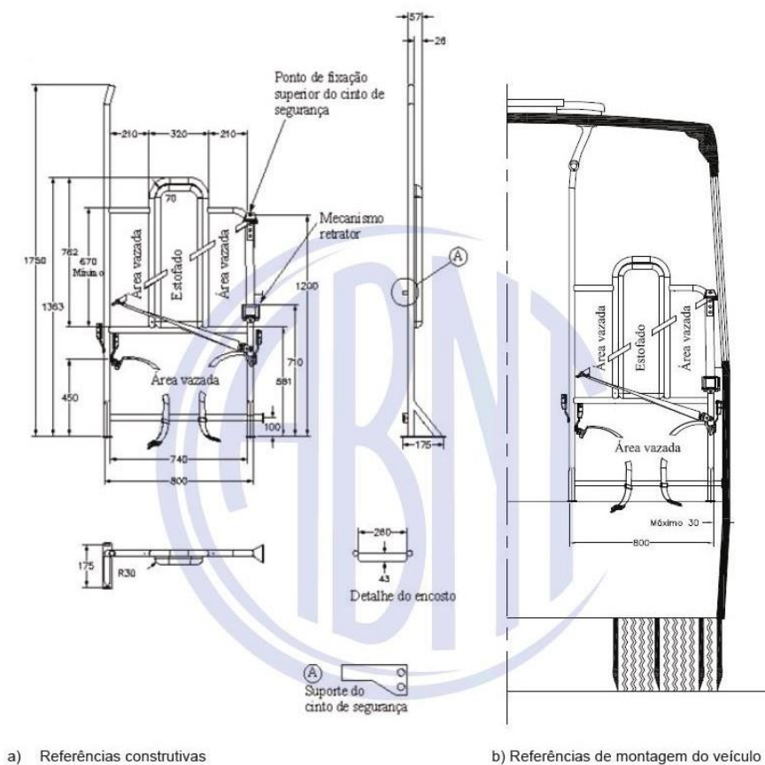
Figura 4 – Referências dimensionais para guarda-corpo de fixação da cadeira de rodas.
