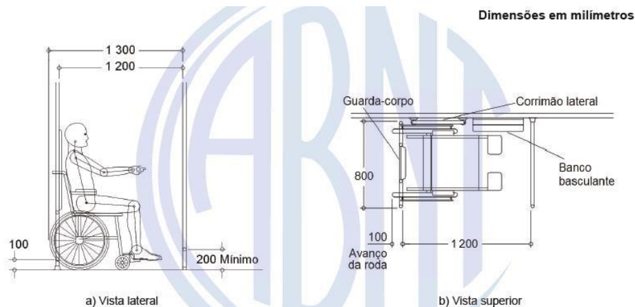
Figura 5 – Referências dimensionais para área reservada.
