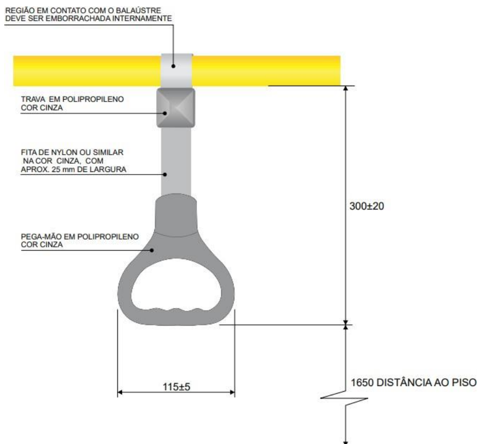
Figura 7 - Detalhe da alça.
