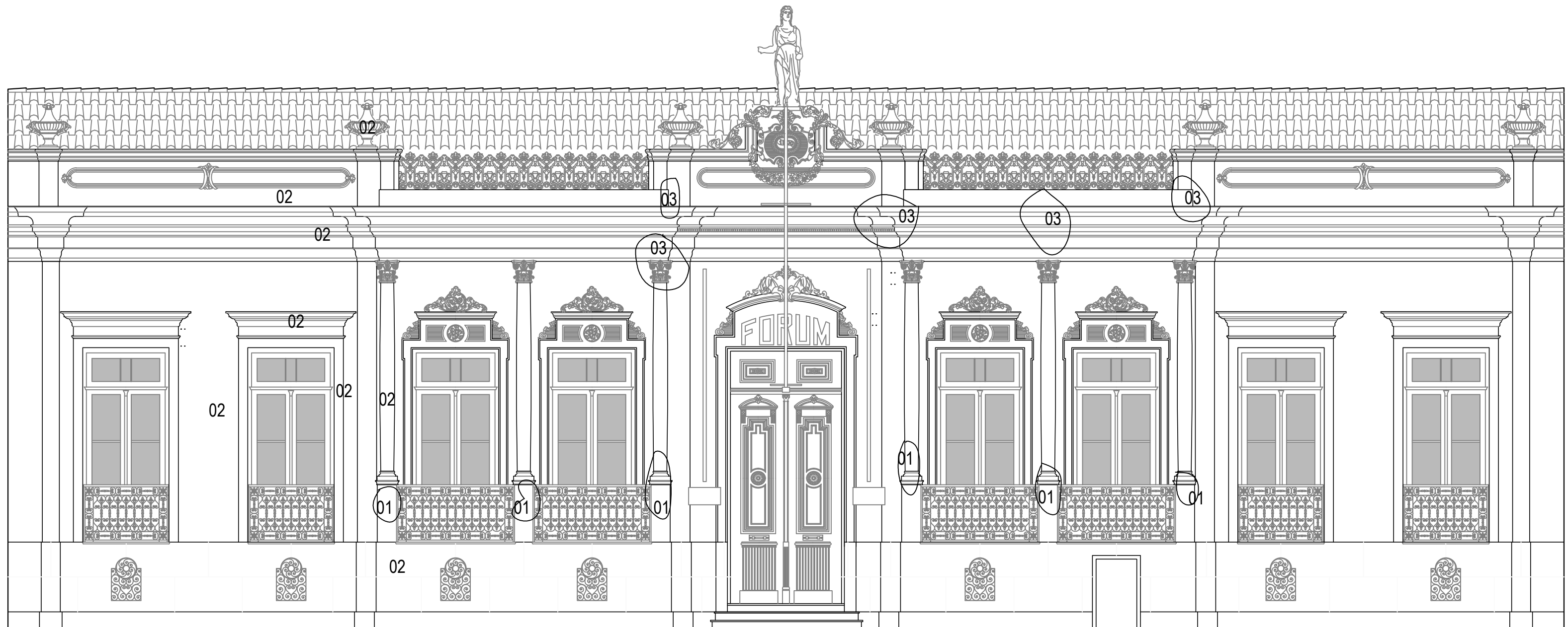
Fachada Principal da Casa de Cultura - Mapa de Danos
