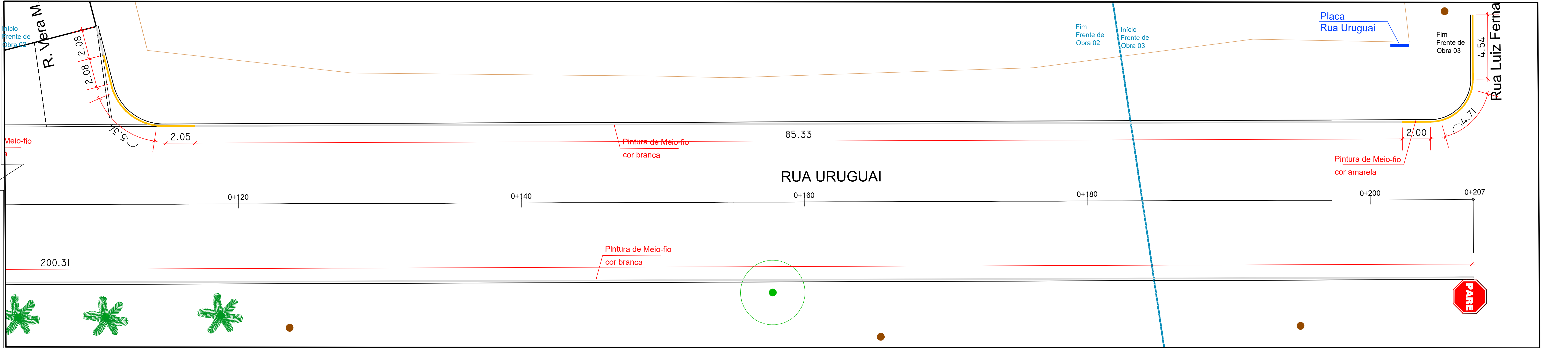
PROJETO SINALIZAÇÃO- Rua Uruguai km 0+105 ao km 0+207 Escala 1:125
