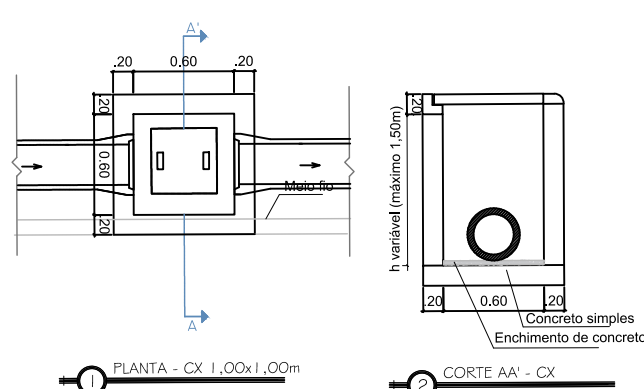
CAIXA DE PASSAGEM 1,00x1,00 (CX N°03/06/13)
