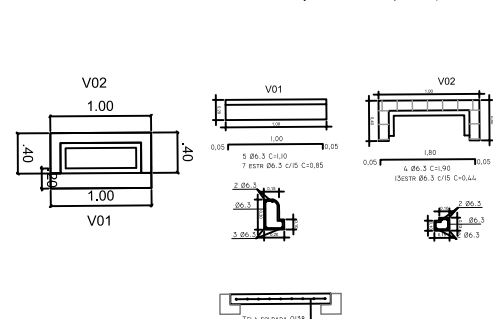
BOCA DE LEÃO (CX N°01/02)
