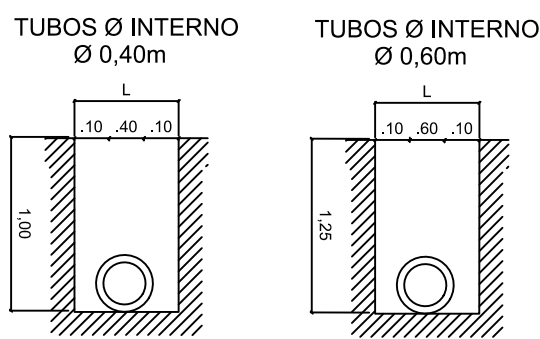
Gabaritos de Escavação
