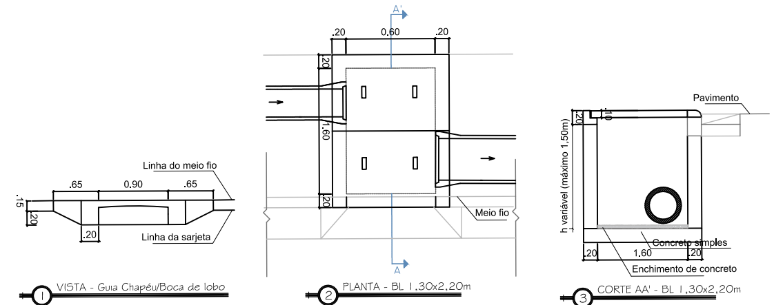
BOCA DE LOBO COMUM 1,00x2,00m (BL N°04)
