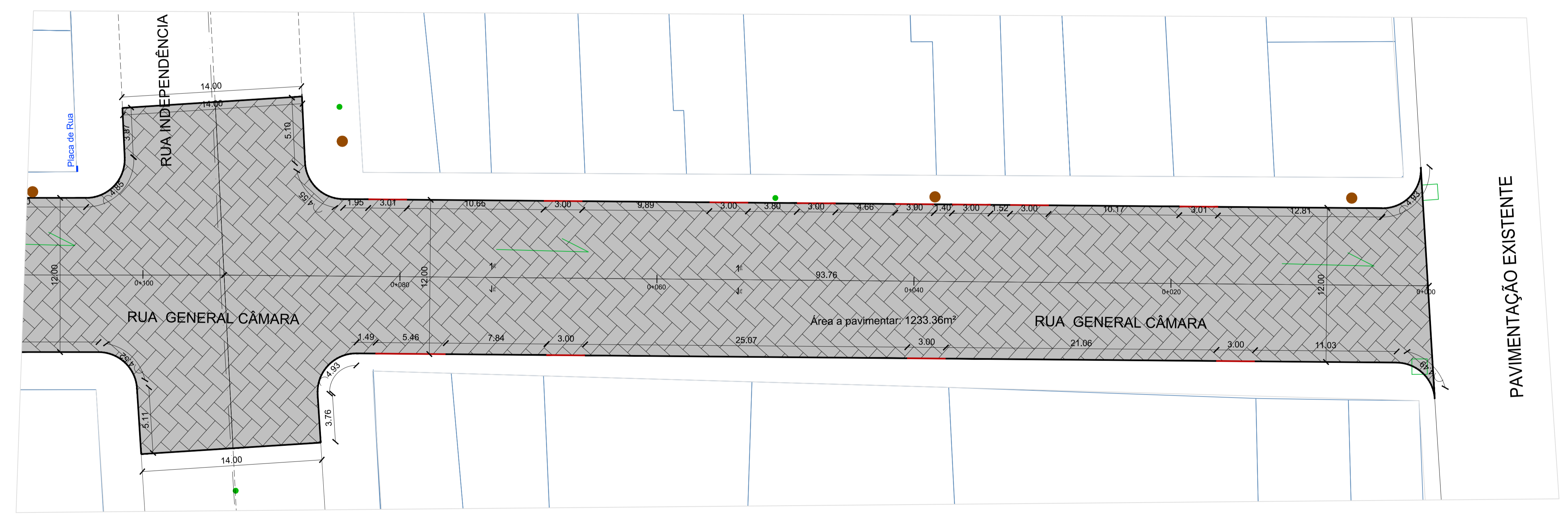
2 Rua General Câmara - Entre Rua Independência e Av. General Bento Gonçalves da Silva ESC: 1:200
