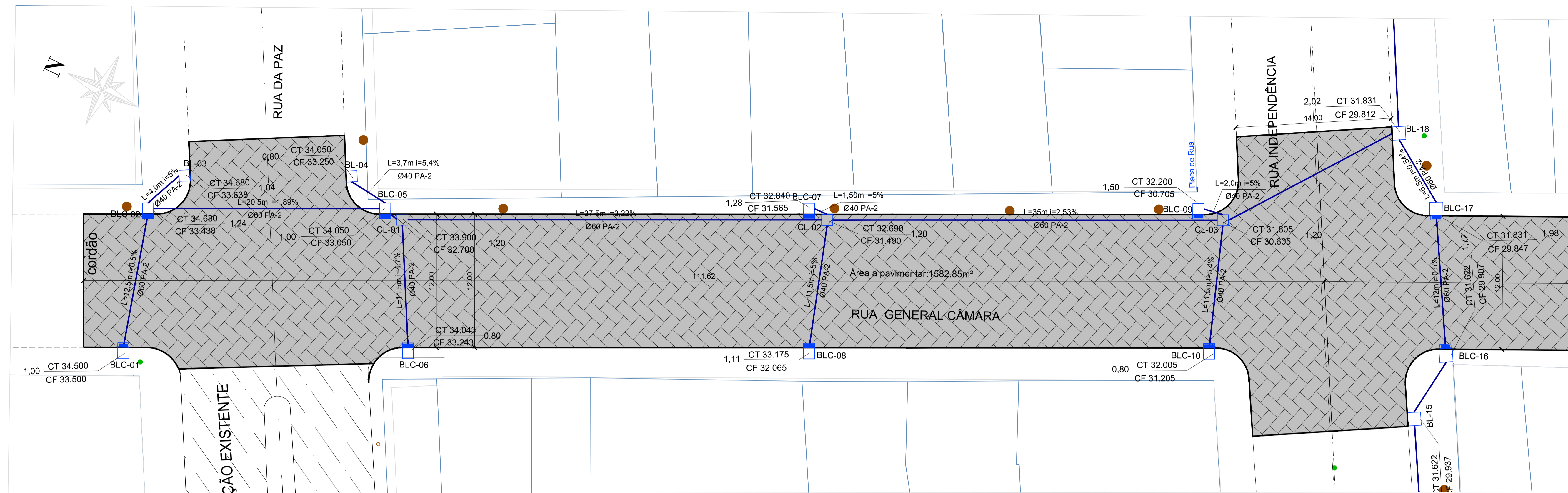
1 Trecho de Drenagem pela Rua General Câmara - Entre Rua da Paz e Rua Independência ESCALA 1:200
