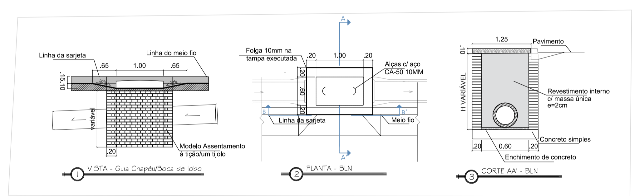
2 Detalhe Boca de Lobo ESCALA 1:50
