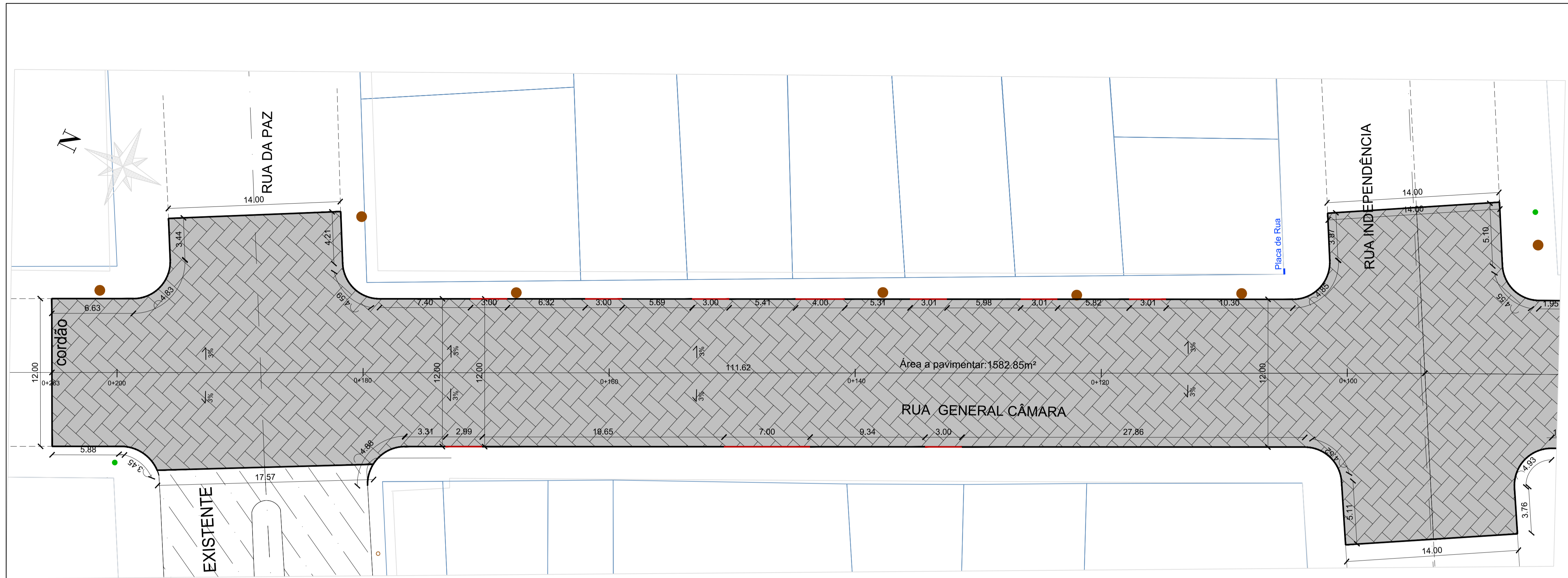
1 Rua General Câmara - Entre Rua da Paz e Rua Independência ESC: 1:200
