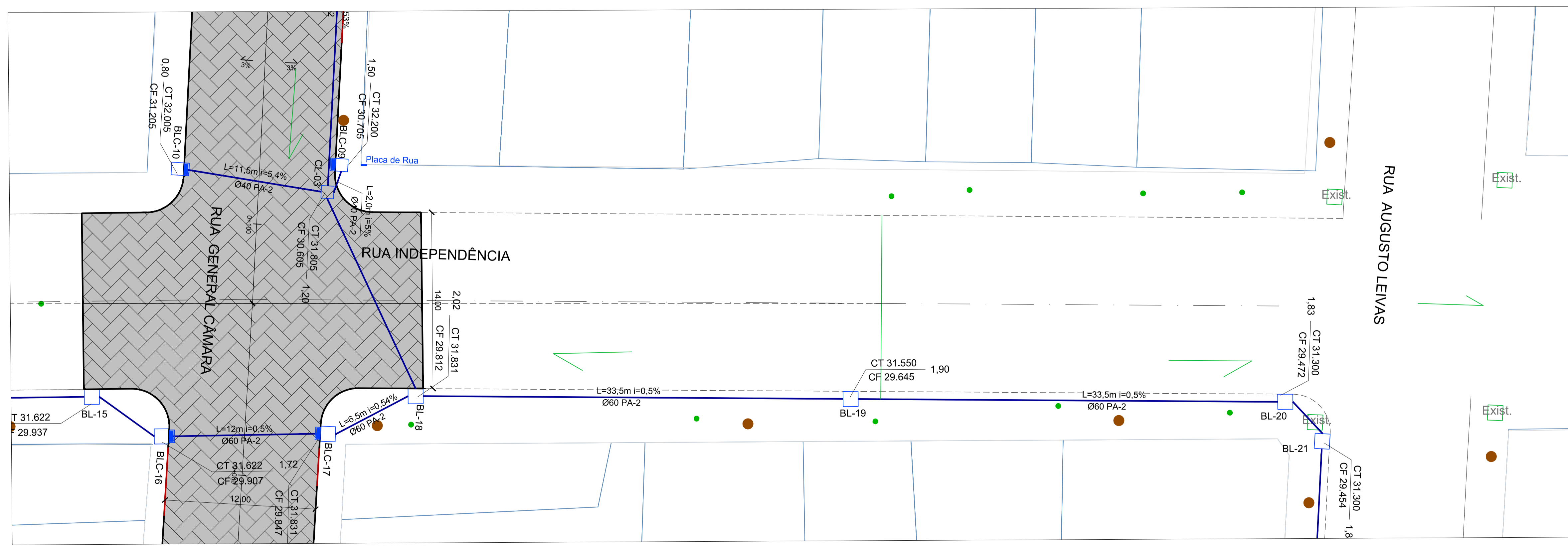
2 Trecho de Drenagem pela Rua Independência - Entre Rua General Câmara e Rua Augusto Leivas ESCALA 1:200
