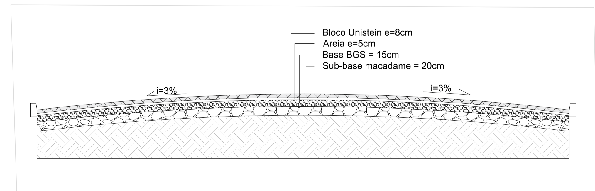
3 Seção Transversal - Rua General Câmara entre Rua da Paz e Av. General Bento Gonçalves da Silva ESCALA 1:50
