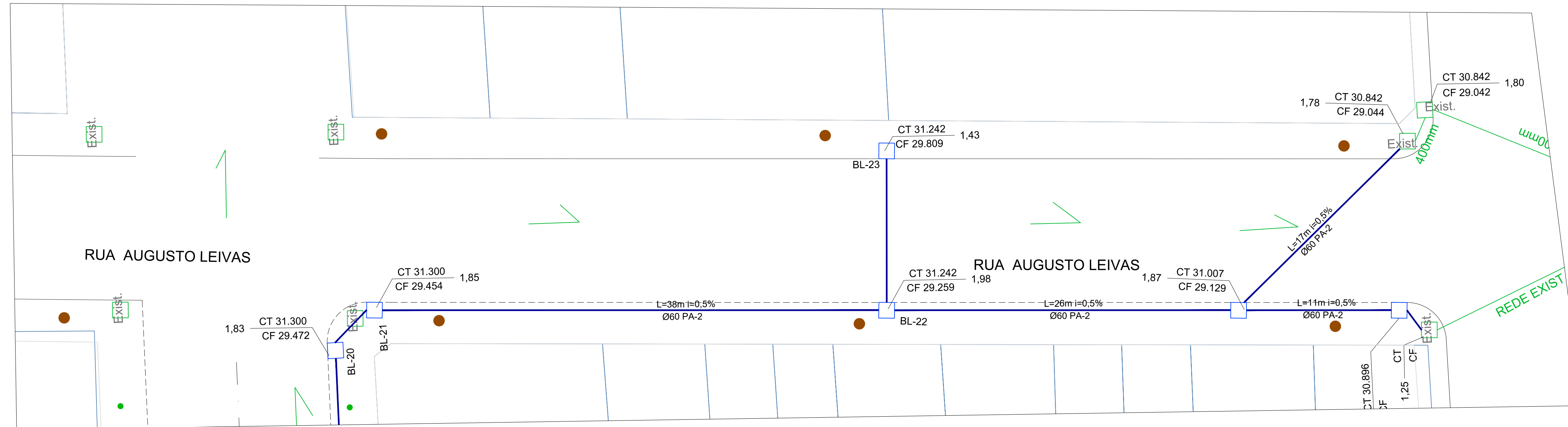
1 Trecho de Drenagem pela Rua Augusto Leivas - Entre Rua Independência e Av. General Bento Gonçalves Silva ESCALA 1:200
