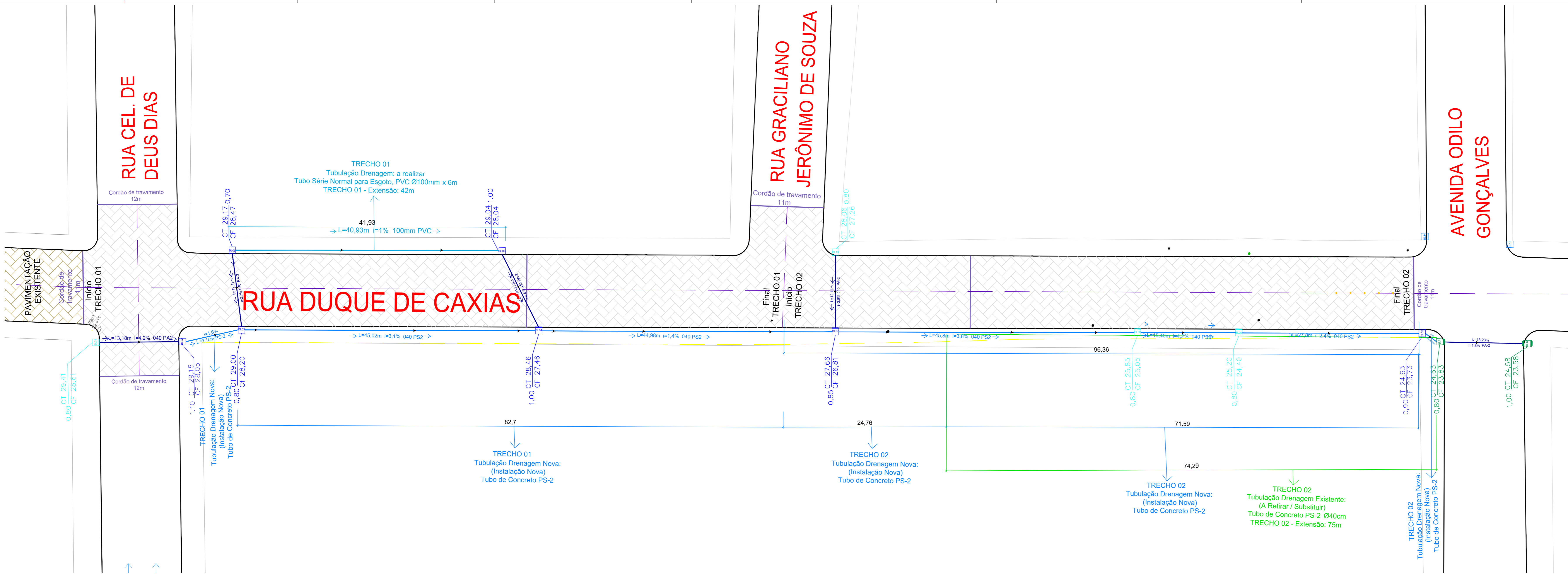
PROJETO DE DRENAGEM- Trecho 01 e 02 - Rua Duque de Caxias (entre Rua Cel. de Deus Dias e Avenida Odilo Gonçalves)
