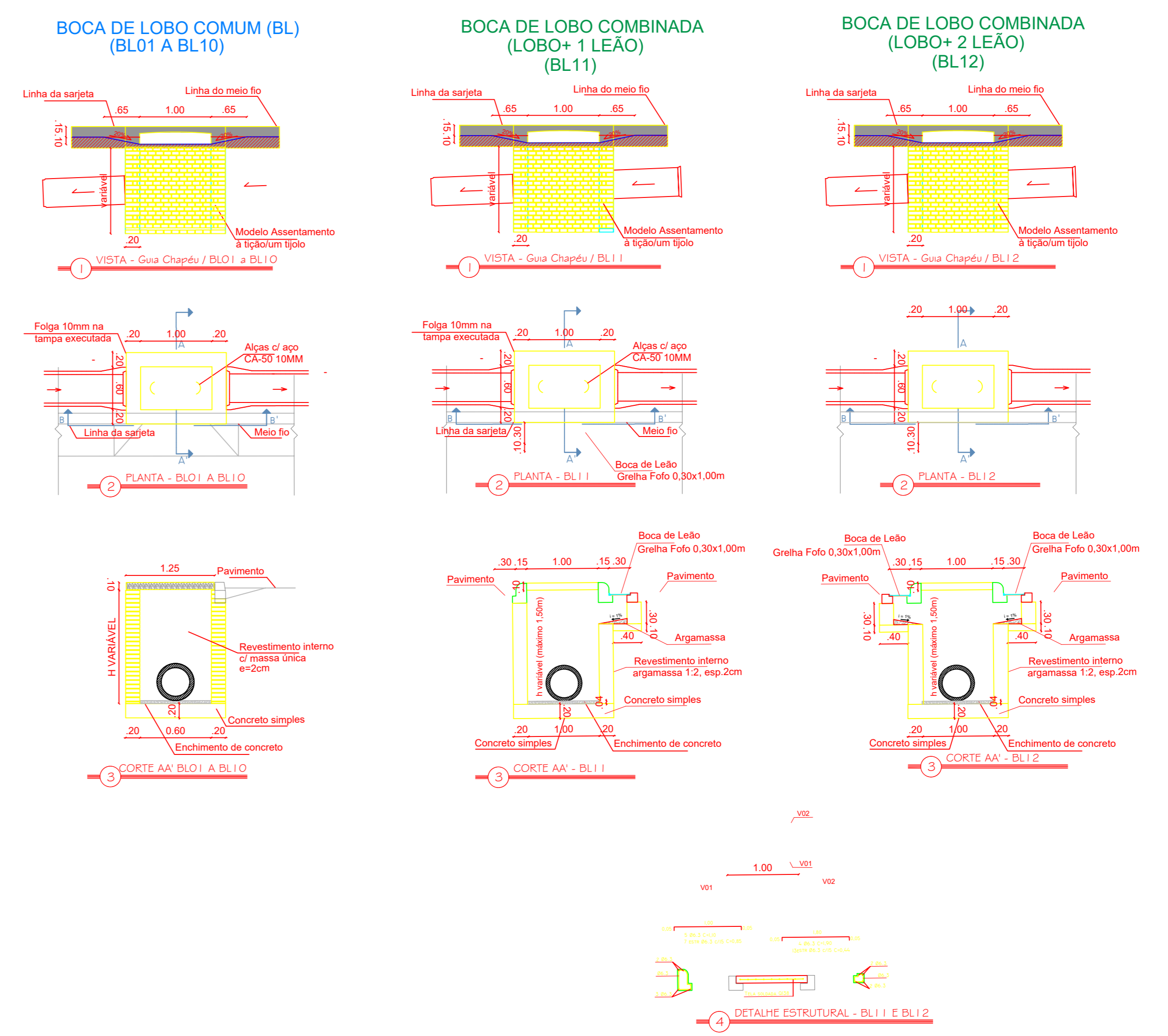
BOCA DE LOBO COMUM (BL01 a BL10) e BOCA DE LOBO COMBINADA (BL11 e BL12)
