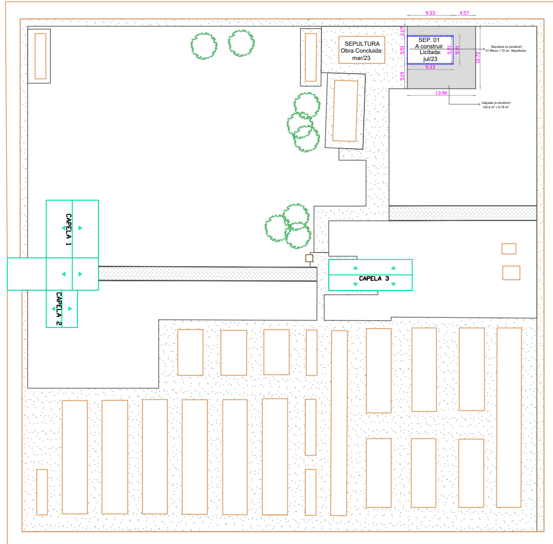
PLANTA SITUAÇÃO- Cemitério Municipal de Jaguarão/RS 1:750
