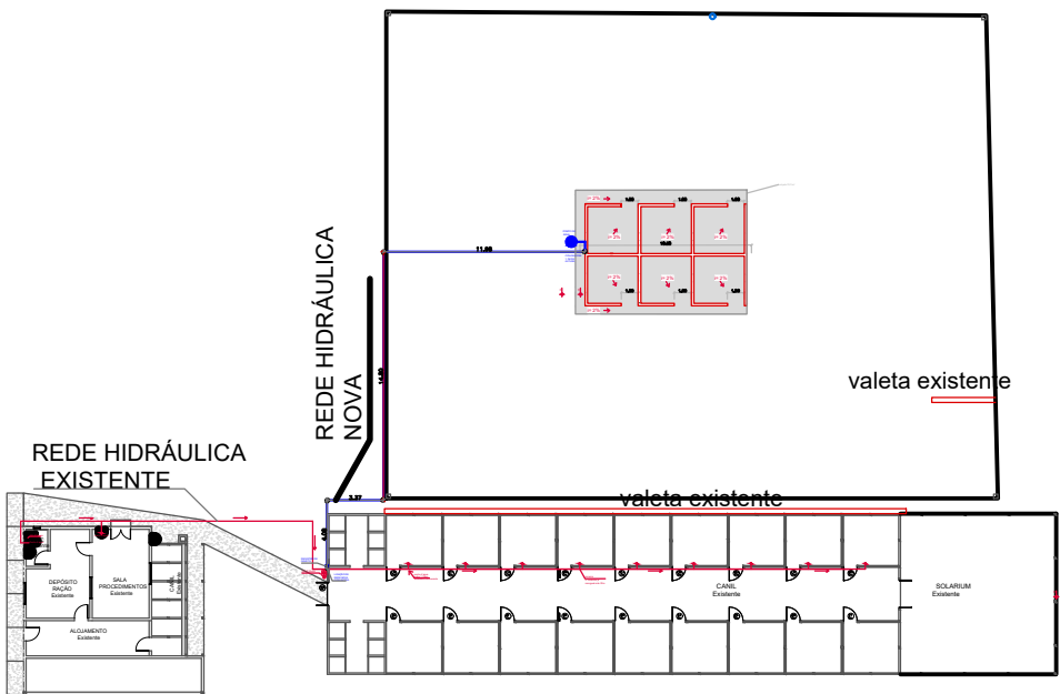
PROJETO HIDRÁULICO ESCALA 1:500
