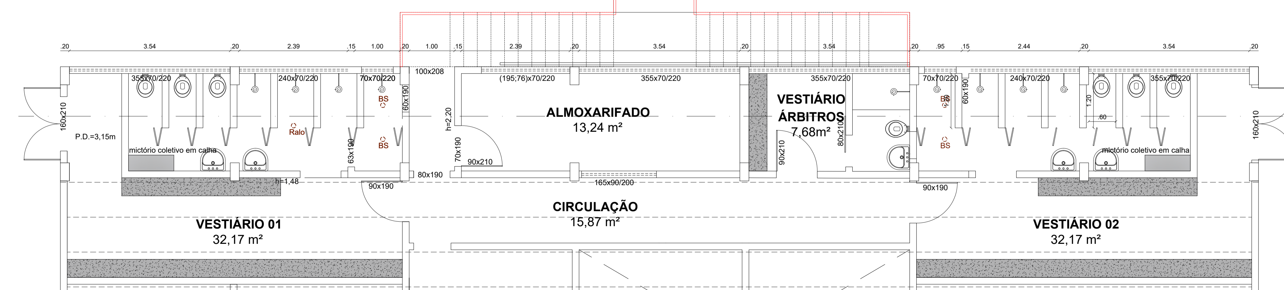
03 PLANTA BAIXA - Final Escala: 1/50
