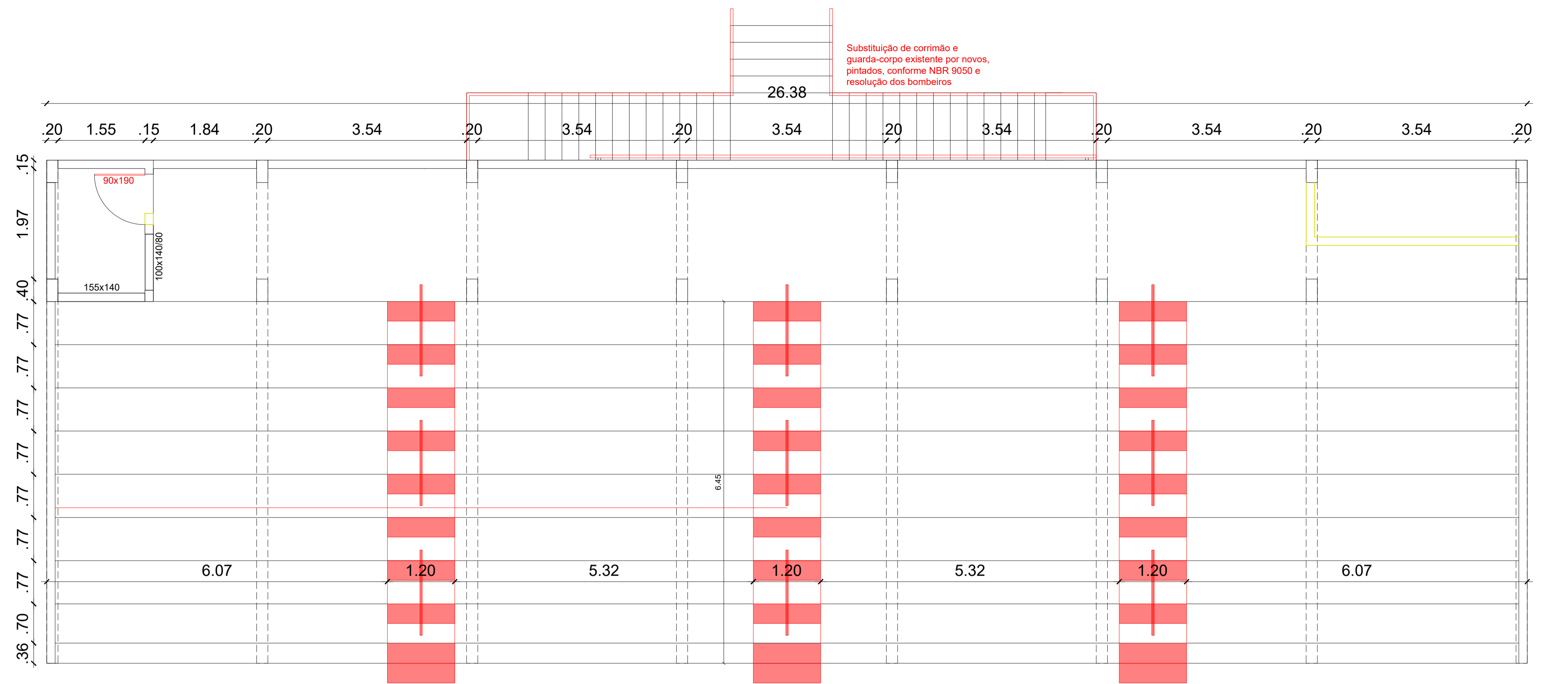
01 PLANTA BAIXA - Demolir/Construir - Arquibancada Escala: 1/50
