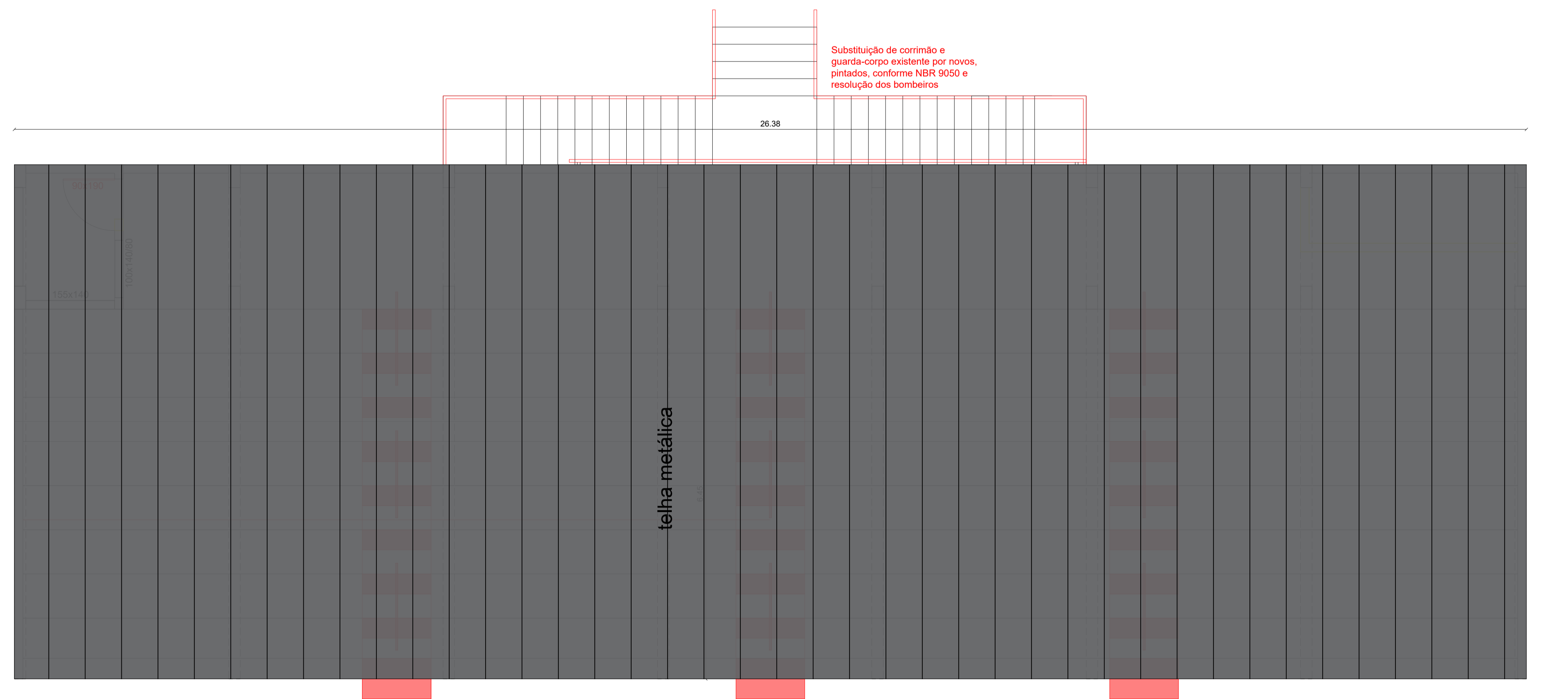
03 PLANTA DE COBERTURA - Final Escala: 1/50
