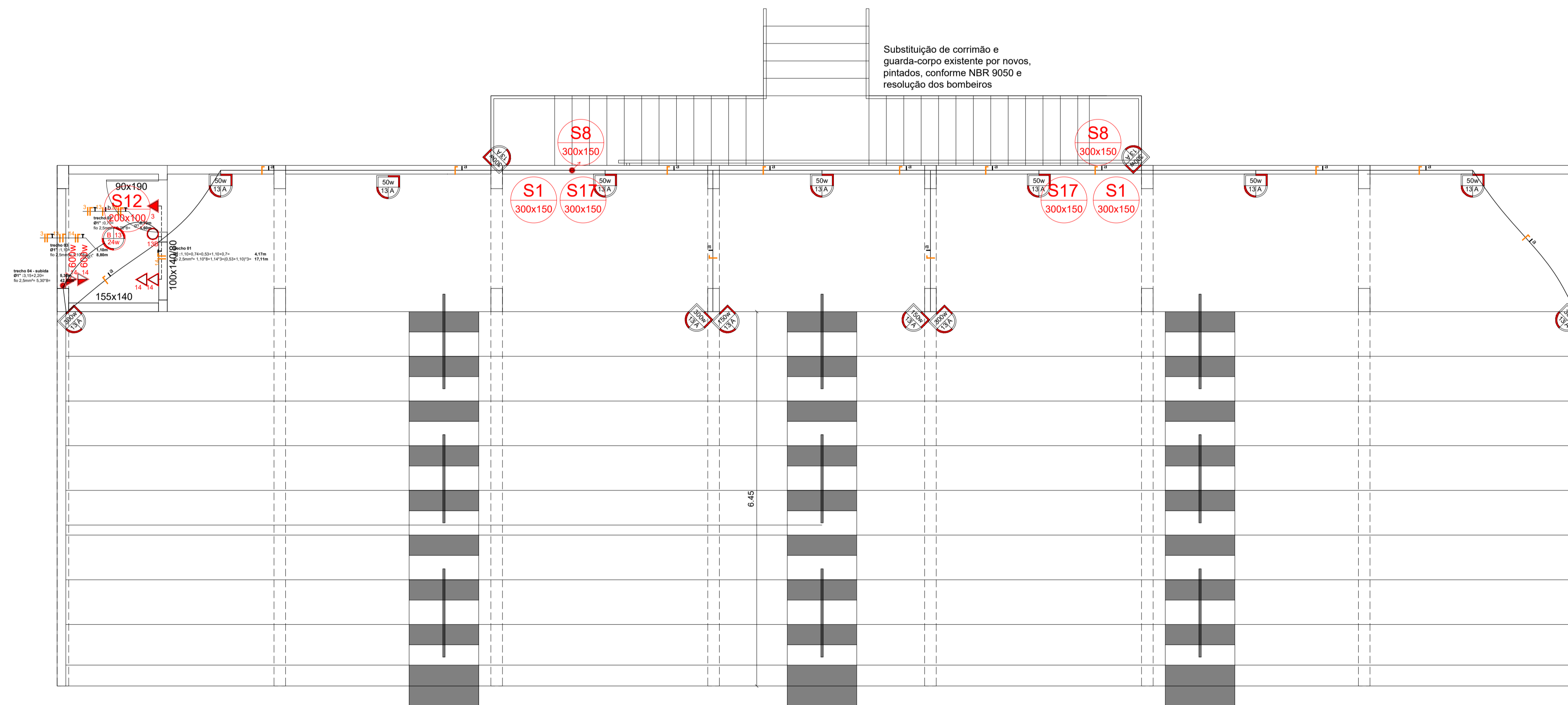
02 PROJETO ELÉTRICO - Arquibancada Escala: 1/50
