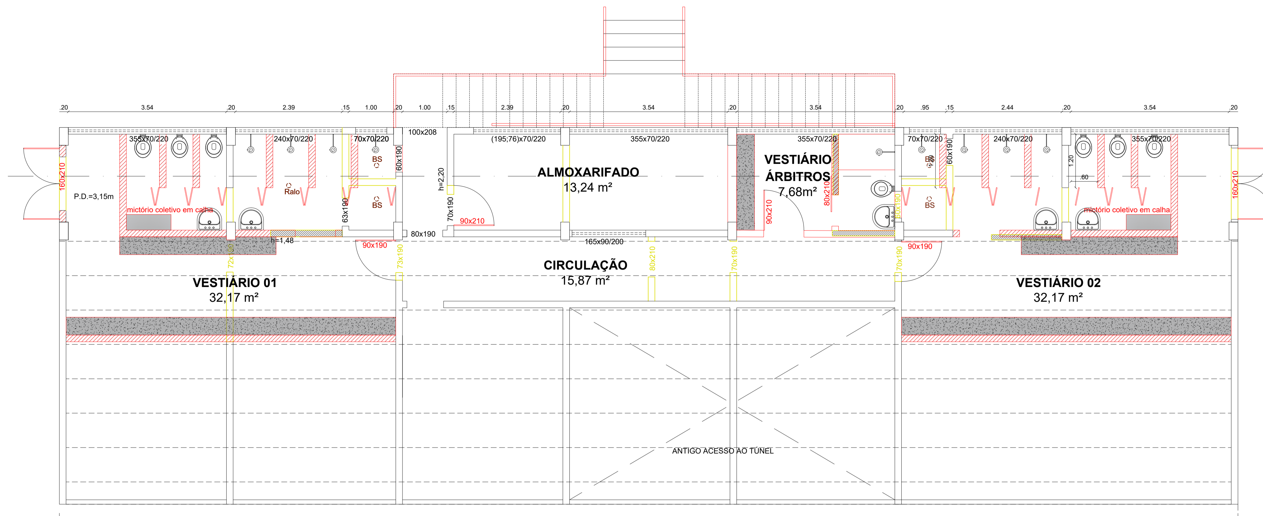
01 PLANTA BAIXA - Demolir/Construir Escala: 1/50
