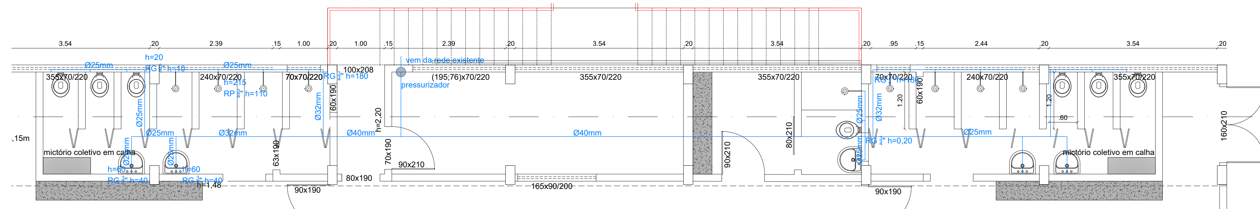
01 PROJETO ESGOTO SANITÁRIO - Vestiários Escala: 1/50
